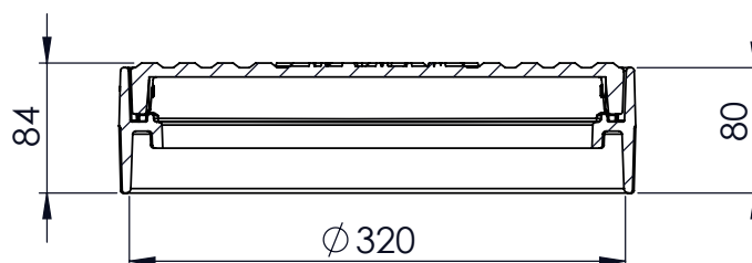
Doorsnede A-A
