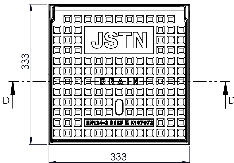
Bovenaanzicht
